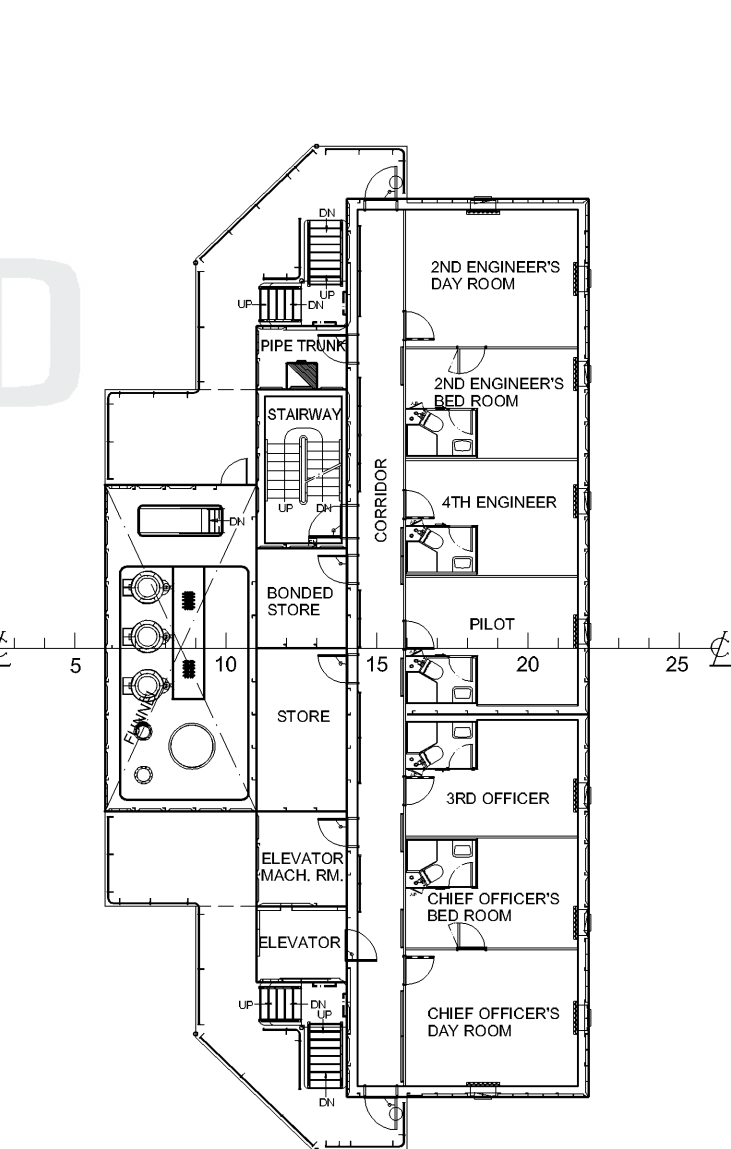
E - DECK
